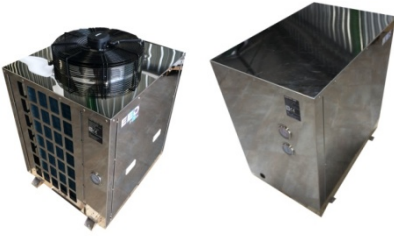
Pompe à chaleur Inox Très haute température 80°C Groupe extérieur + intérieur
